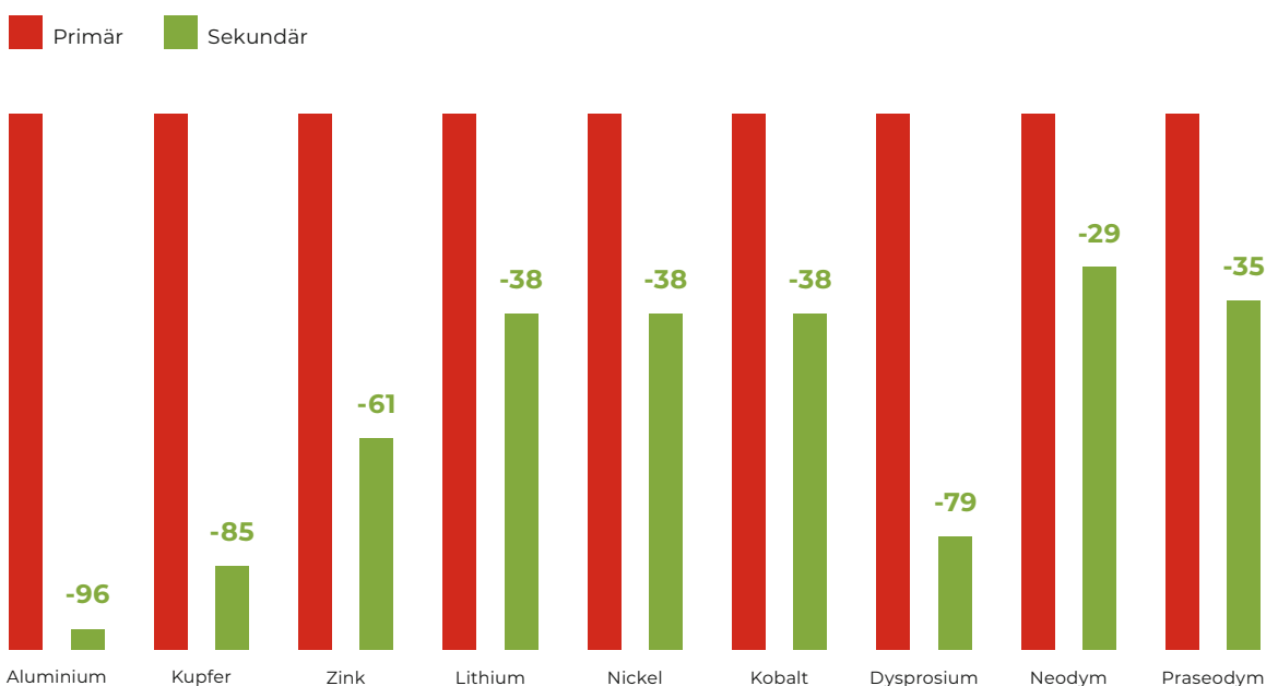
Abbildung 5 – CO 2 Einsparungen (in %) von Metallen und ihren Rezyklaten im Vergleich
