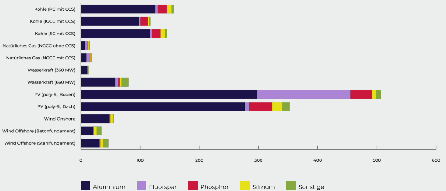
Abbildung 2 – Bedarf an kritischen Rohstoffen für ausgewählte Energietechnologien in g pro MWh
