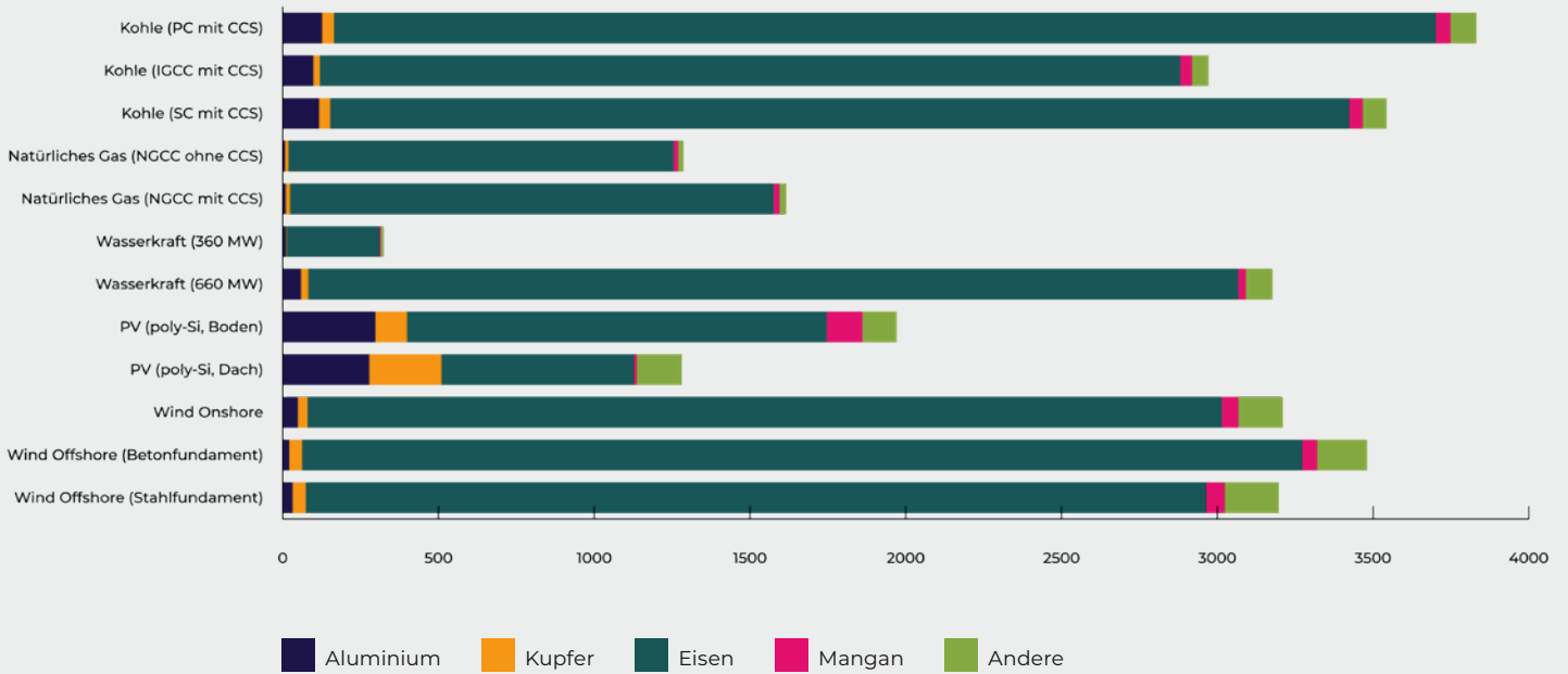
Abbildung 1 – Metallbedarf für ausgewählte Energietechnologien in g pro MWh
